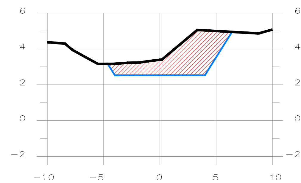
SECCION 5+434.55
