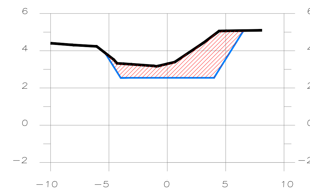
SECCION 5+454.55
