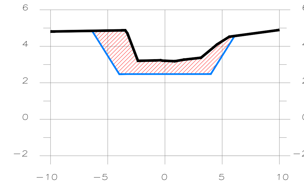
SECCION 5+374.55
