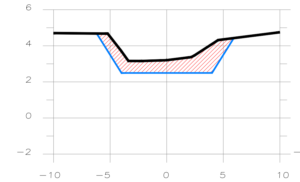
SECCION 5+394.55
