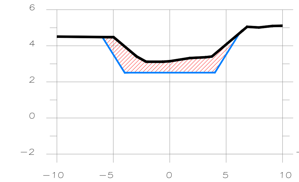
SECCION 5+414.55
