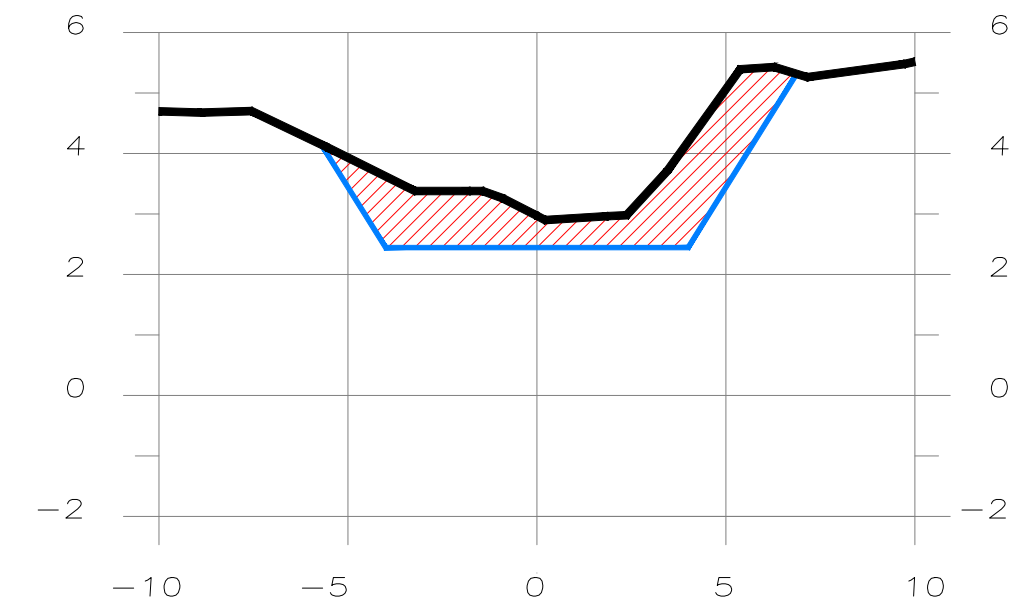
SECCION 5+334.55
